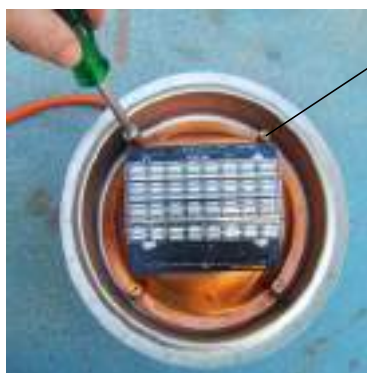
Tuerca de retención (4x)
